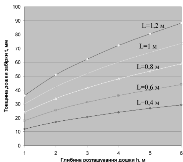
Рис. 7. Графік залежності товщини дощок забірки від кроку стояків та глибини її розташування, коли ґрунт знаходиться в водонасиченому стані
